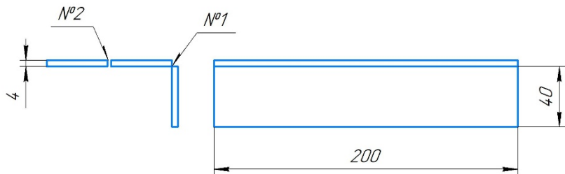
КСУ №1 стыковое и угловое соединение по ГОСТ 5264-80
